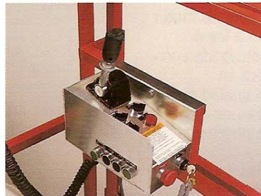
La palanca universal de control permite a los trabajadores realizar todas las funciones desde la plataforma. Se puede retirar para evitar el uso no autorizado.
